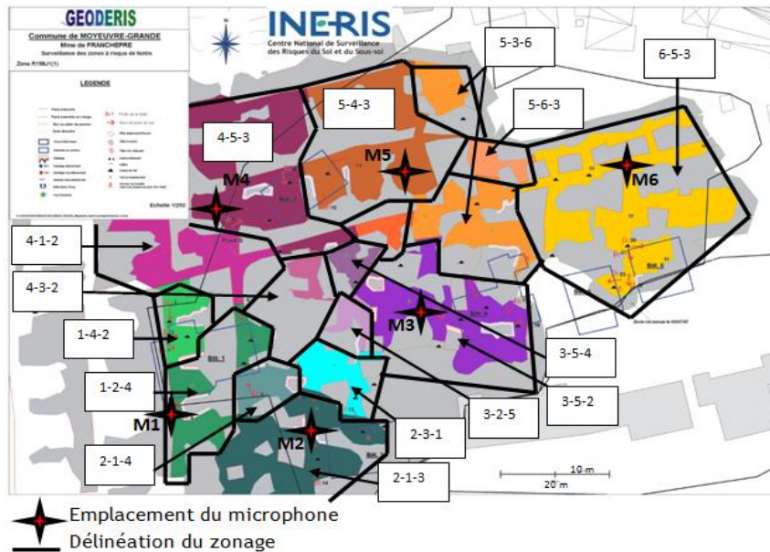
Figure 3. Zonage des premiers temps d'arrivées aux capteurs déterminé par des tirs au pistolet d'alarme. Pour chaque zone, les 3 capteurs déclenchés en premier sont indiqués.
