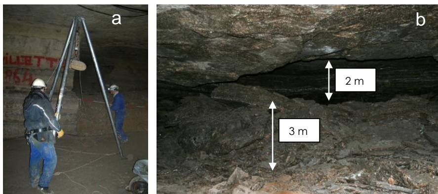
Figure 2. a : Simulation de chutes de bloc de calcaire dans une carrière abandonnée en région parisienne. b : Chute de toit évaluée à 200 tonnes enregistrée par le réseau de surveillance acoustique en place.
