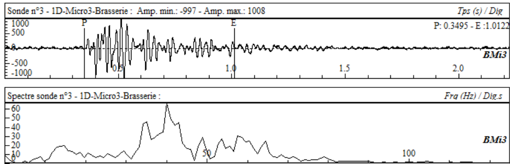
Figure 1. Signal acoustique enregistré par l'INERIS lié à une chute de bloc dans une carrière de calcaire de région parisienne (pression acoustique et enveloppe spectrale).
