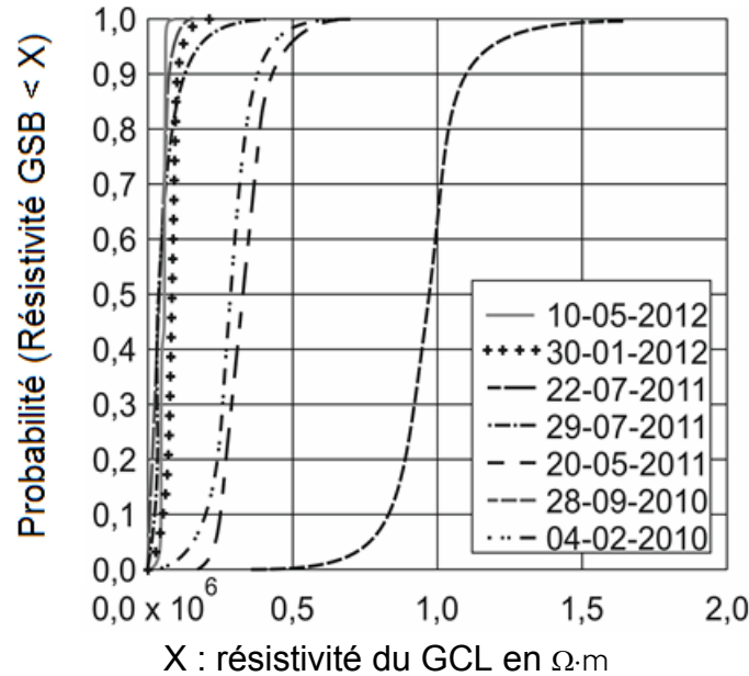
Figure 3. Distribution des valeurs des résistivités électriques ( \Omega \cdot m en abscisses) du GSB obtenues par la méthode des essais particuliers (fréquences cumulées en ordonnées).
